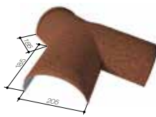
TRÓJNIK GAŚIORA 205 15-30°
