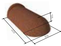
GAŚIOR POCZĄTKOWY 205
